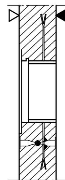
Coupe A-A
