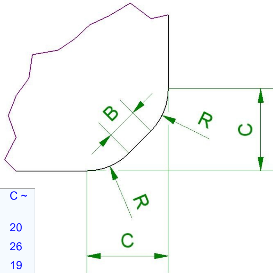
Géométrie du chanfrein des colonnes carrées centrifugées
